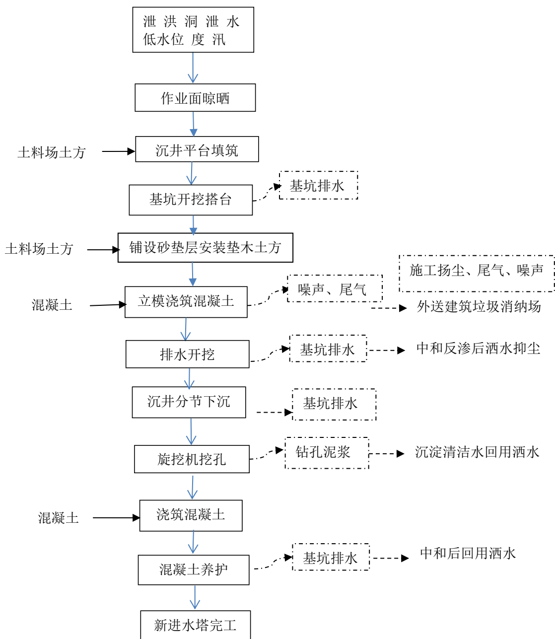
图 4.3-6 新进水塔施工流程及影响节点图
