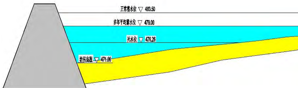
图 4.4-1 洹河水库水位特征值示意图
