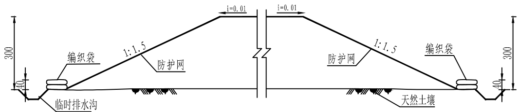
A-A 剖面图 1:100
