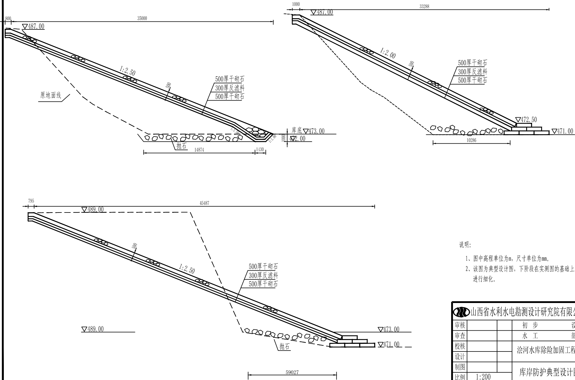
附图4-3 库岸防护典型设计图
