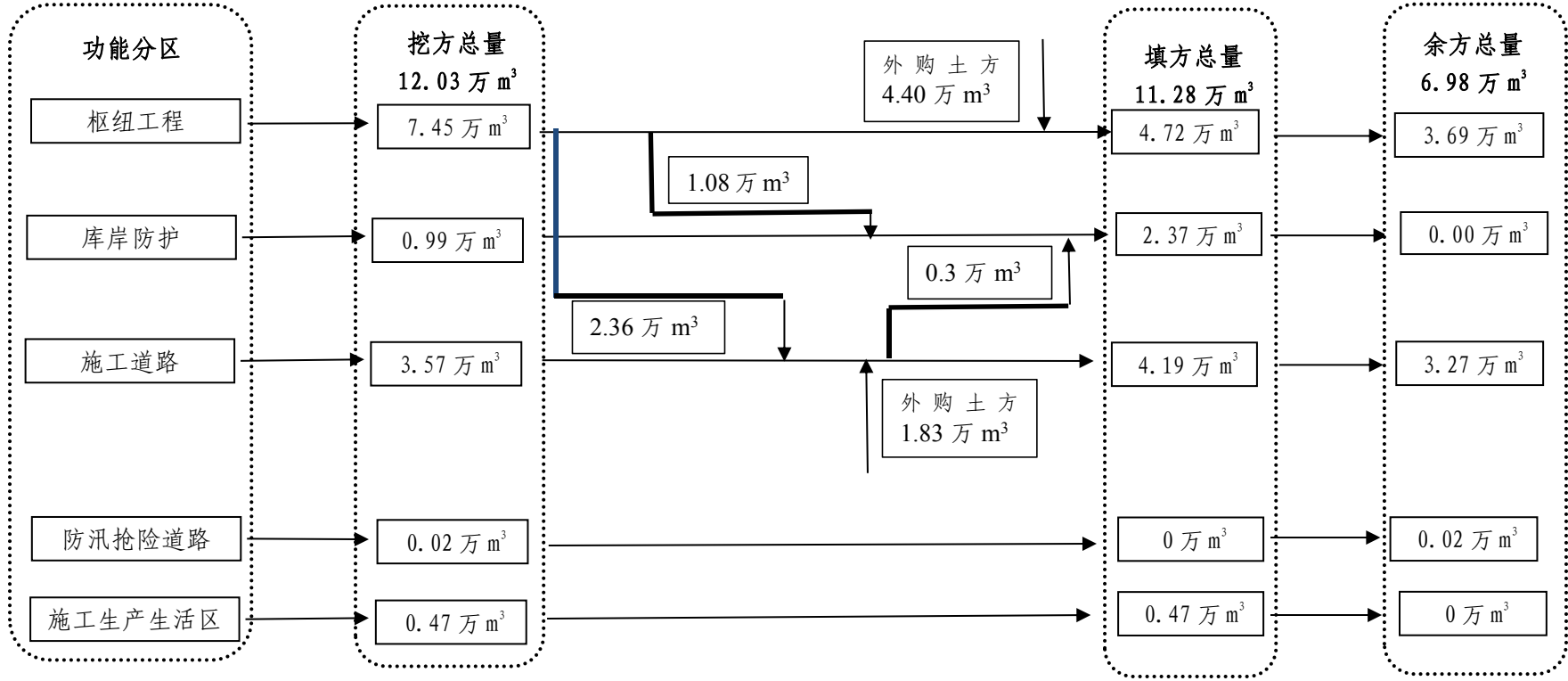
图 3.2-6 土石方流向框图
