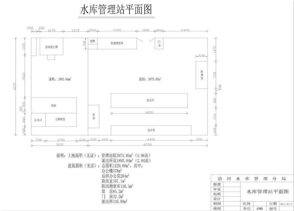
图 3.1-6（2） 管理站平面布置图
