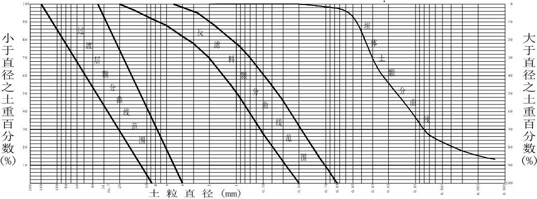
颗粒大小分配曲线
