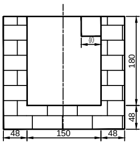
B—B剖面图 1:50
