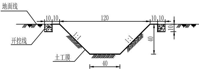
临时排水沟剖面图 1:20
