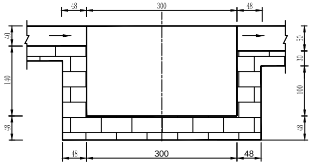
A—A剖面图 1:50
