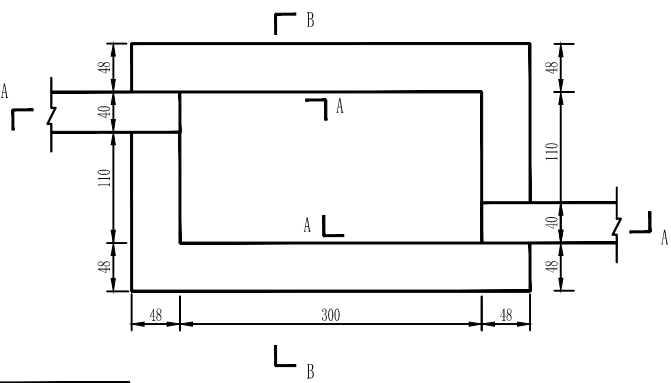
临时堆土场沉砂池平面布置图 1:50
