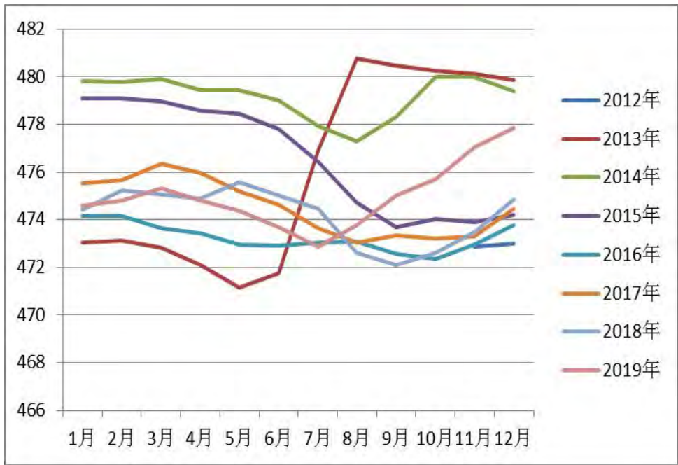
图 6.1-3 浍河水库 2012~2019 年水位变化过程图
