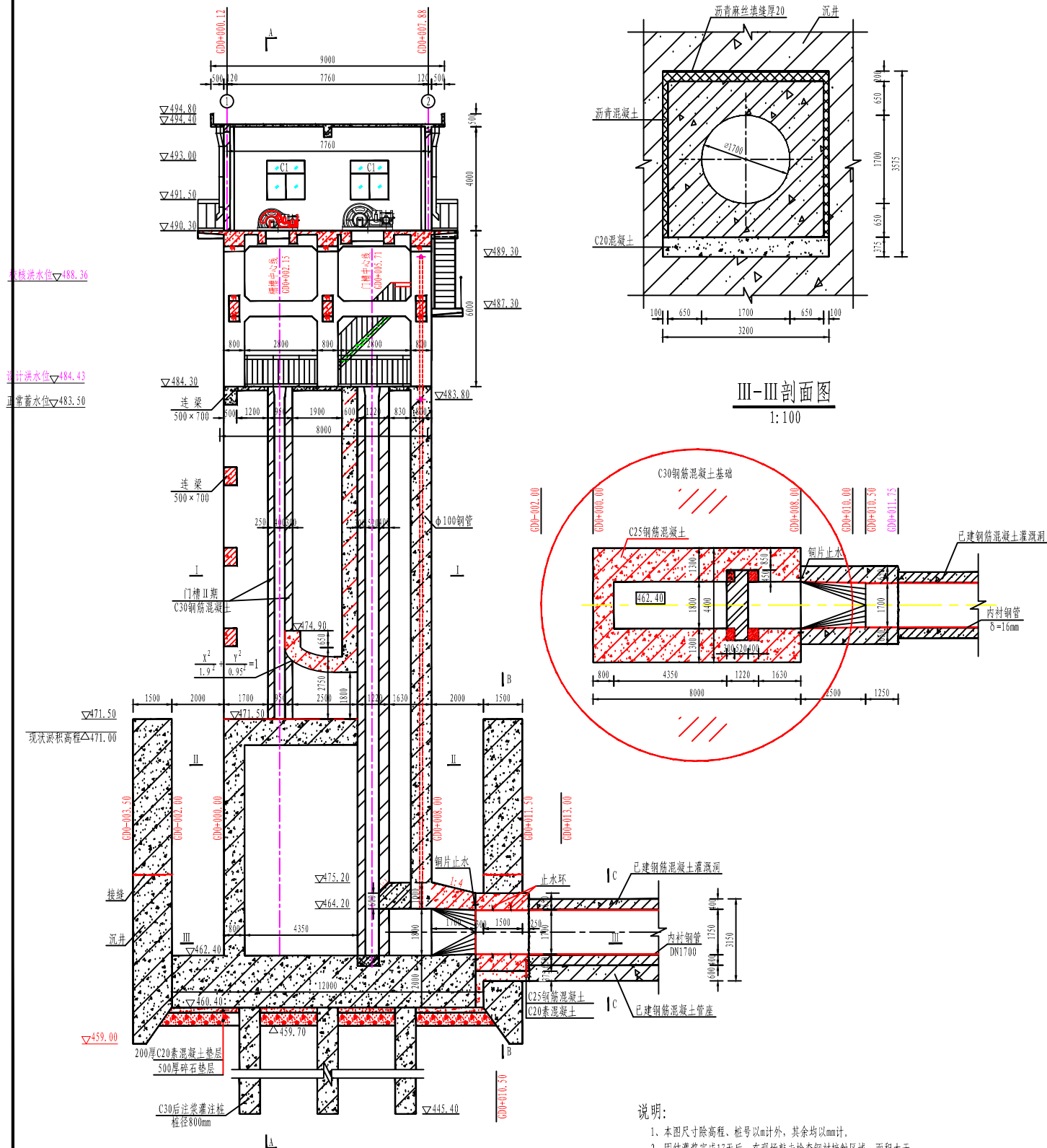
B-B剖面图
