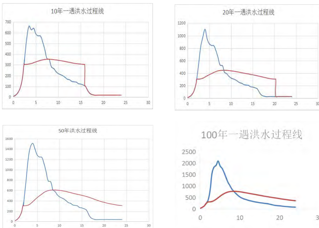
图 6.1-4 洪水过程线形态变化图
